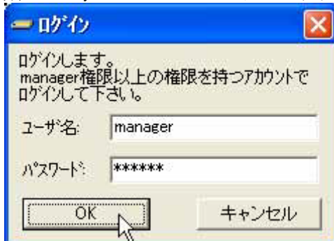
図3.3.7 ログイン
